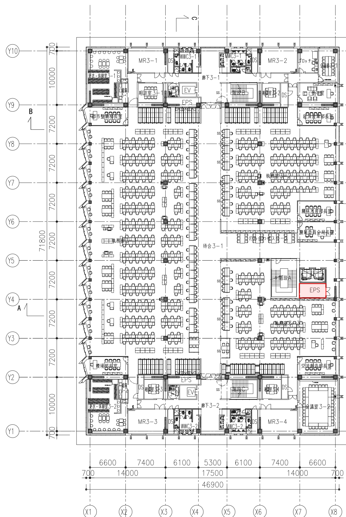
3階平面図（建築基準法上4階）
