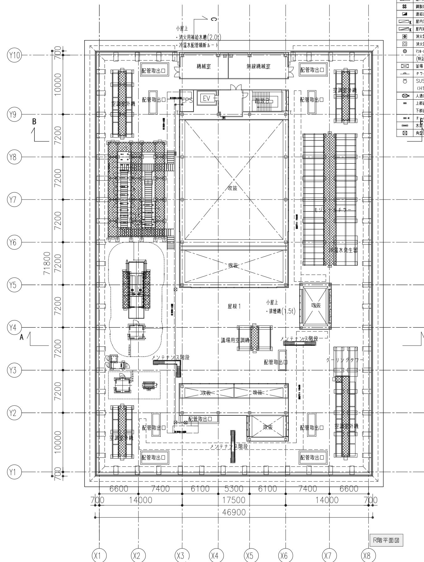
6階平面図 (建築基準法上7階)
