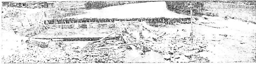
上の写真は大字路筋高瀬橋工事、工事模様で、延長54mのコンクリート橋、5月30日完工予定です。
