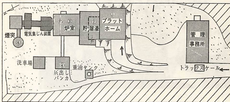
清掃工場配置図
