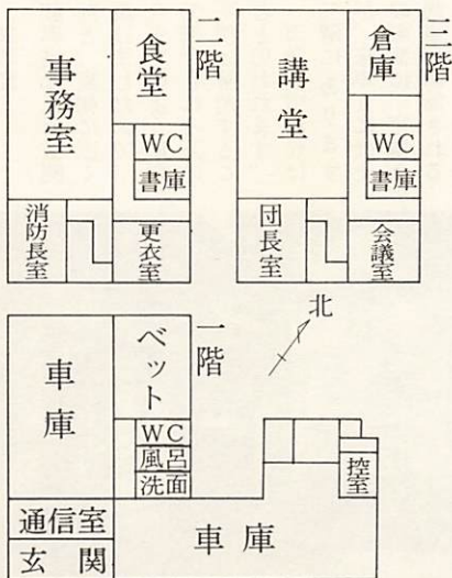
消防庁舎配置図
