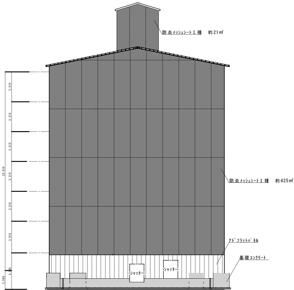
正面立面図案 1/200
