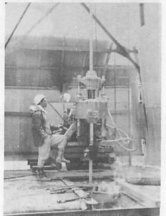
泉源の保護対策として寿泉荘敷地内で進められている泉源掘削工事。現在、300センチまでを掘削。7月には目標の500センチに達する見込みです。
