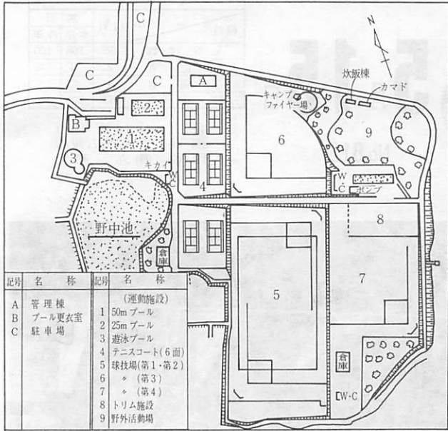
△配置図
