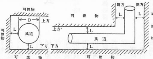
〔設置例〕 液体燃料温風暖房機
