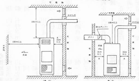
〔機器例〕 液体燃料ストーブ
