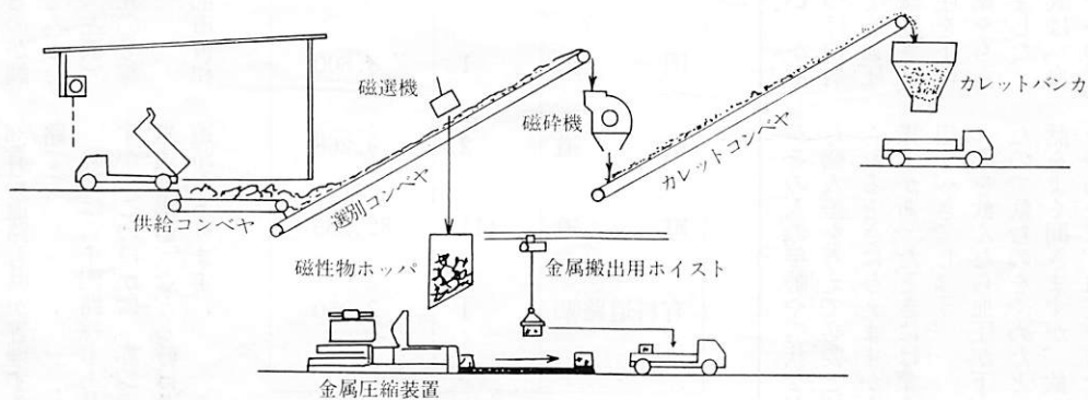
不燃物処理系統図
