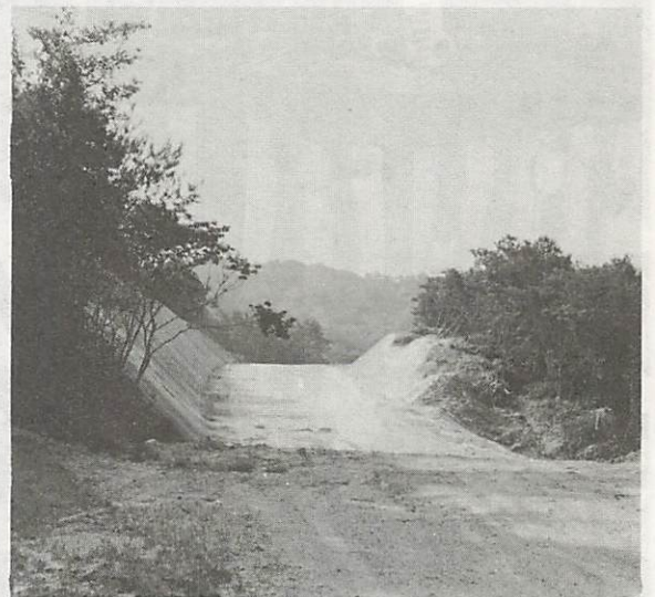
建設が進む、県道山中阿知須線。国道2号から佐山中核工業団地の間は62年度、同団地から国道190号までの間は65年度完成の予定です
