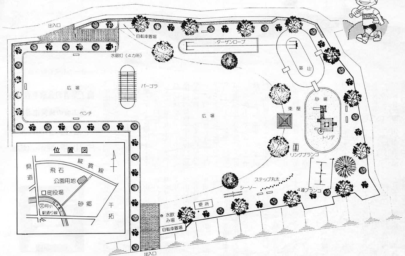
船渡児童公園平面図（案）
