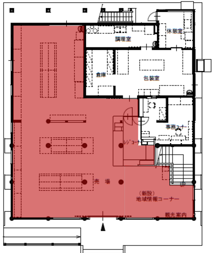
1階平面図（改修後）
