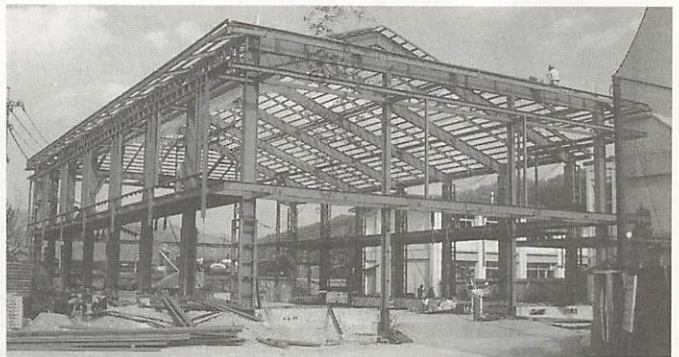
建設中の堀中体育館
