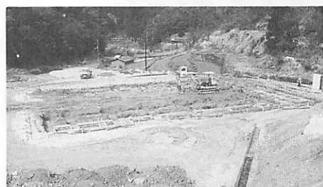
中河内エリアの体験交流センター基礎工事の状況
