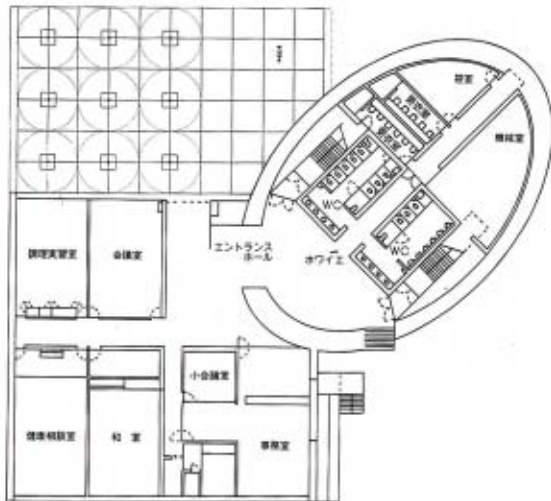
事務所棟1F平面図
