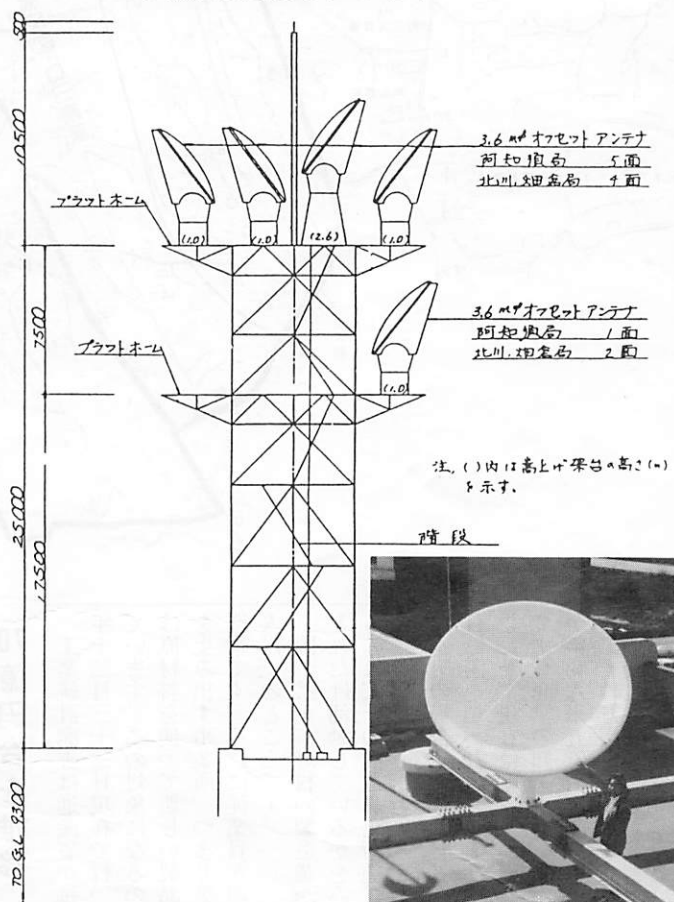
国際電話用のアンテナ
