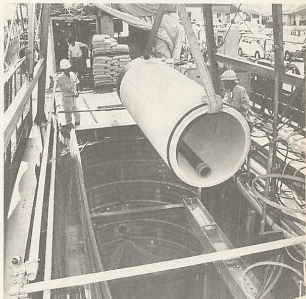
地下8mに管を吊り込む下水道工事(葵一丁目)
