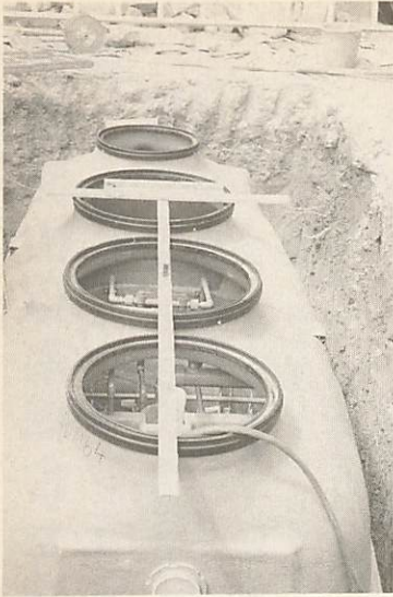
△合併処理浄化槽(8人槽)の埋設工事。ほぼ車1台分のスペースがあれば設置できる。
