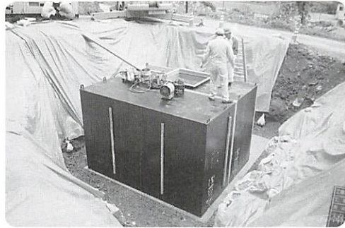
▲耐震性貯水槽の整備
