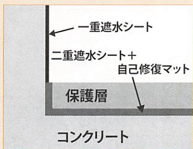
埋め立て施設の構造。コンクリート構造で、底は遮水シートを二重にするなど万全な漏水対策を施します。
