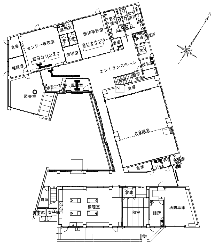
1階平面図
