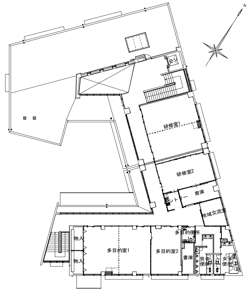
2階平面図
