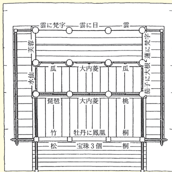
墓股裝飾位置図
