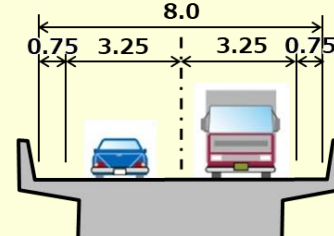
＜橋梁部＞
