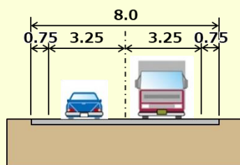
＜標準部＞
