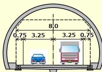
＜トンネル部＞
