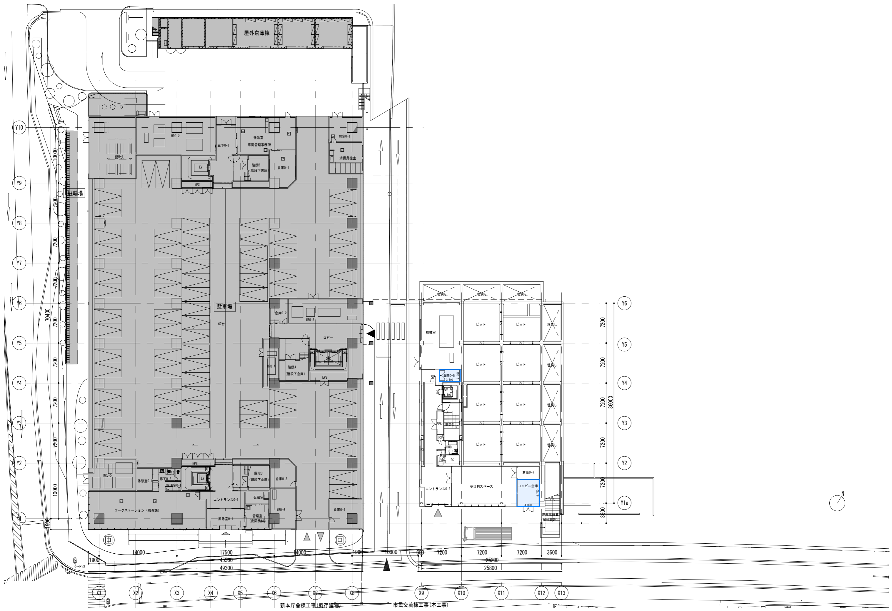
地下1階平面図
