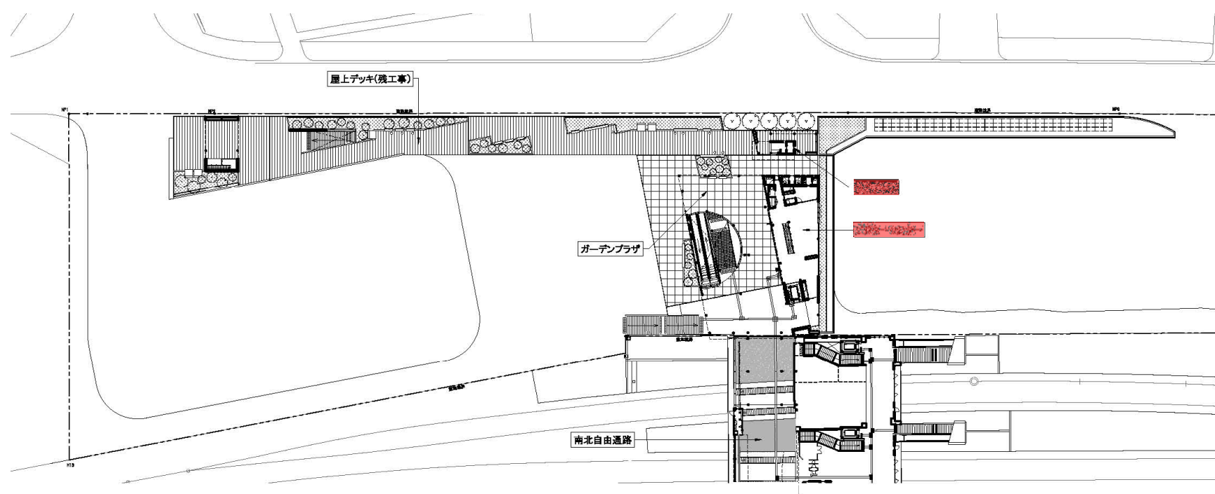
3階平面図
