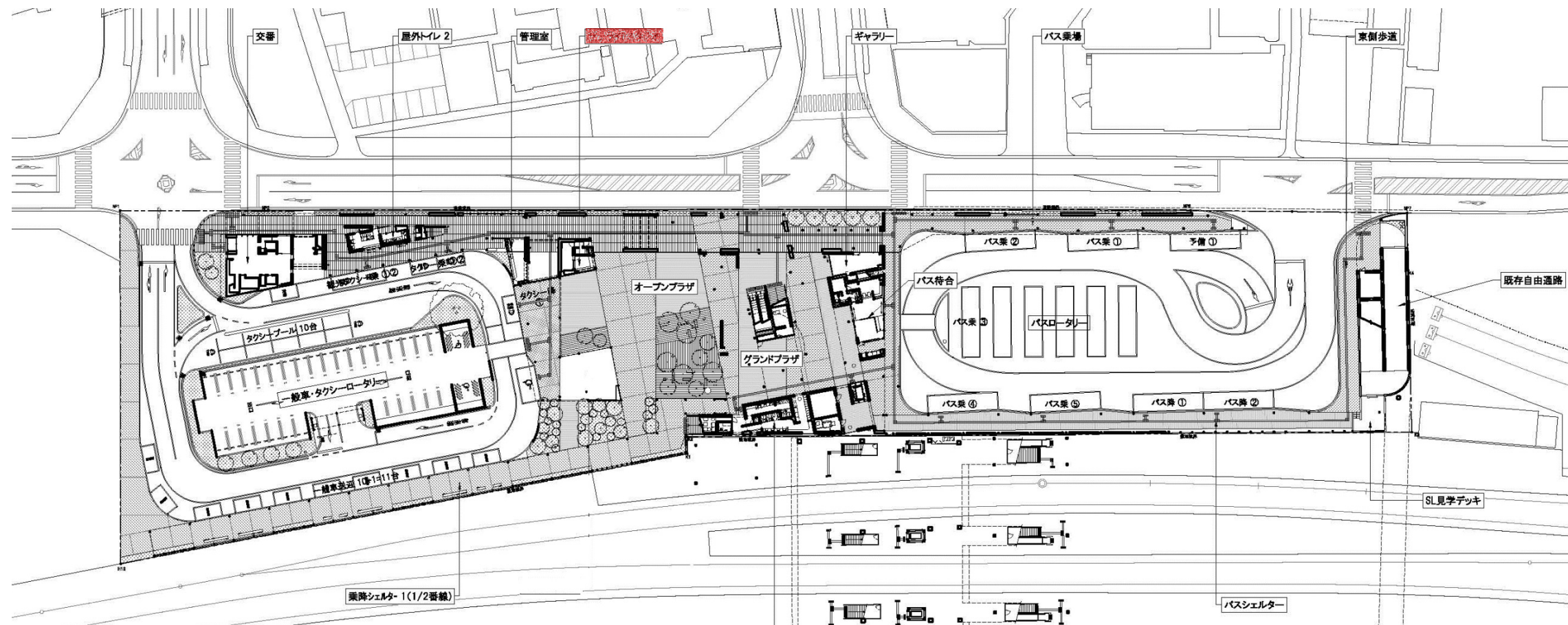
【1階平面図】
