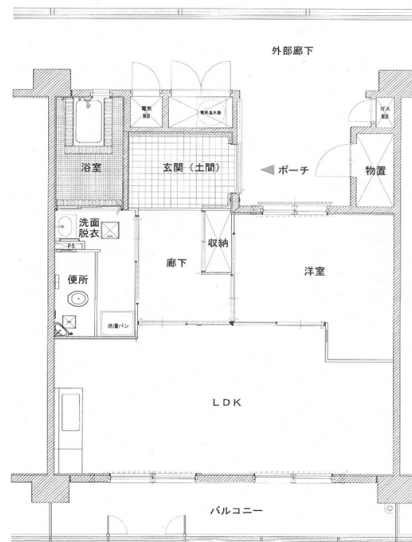
内部平面図
