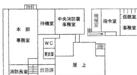
2階平面図
