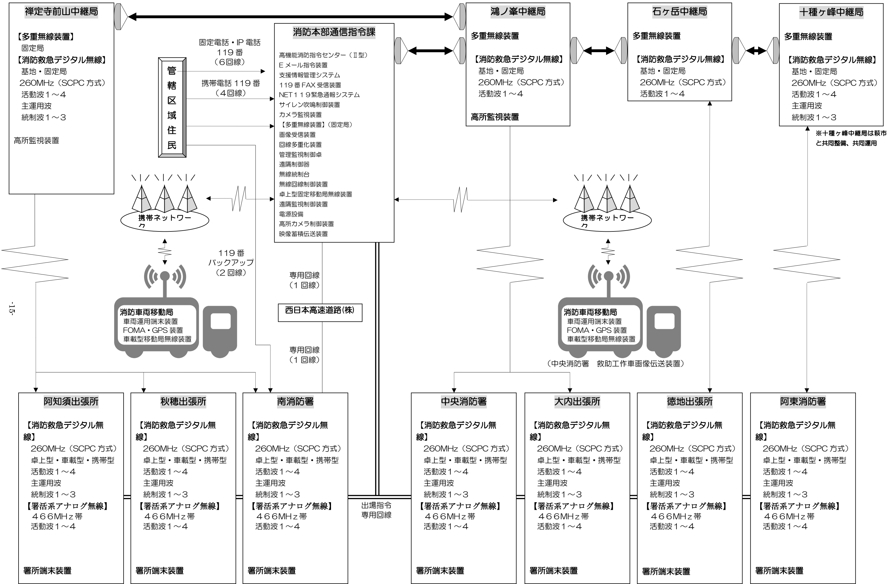
6. 消防通信系統図 (令和7年4月1日現在)
