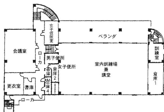
2 階平面図
