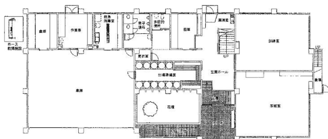
1 階平面図
