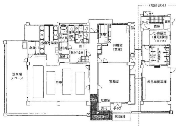
1 階平面図
