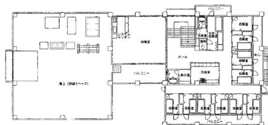
2 階平面図
