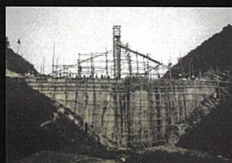
羽根越貯水池堰堤工事 (昭和2年頃)
